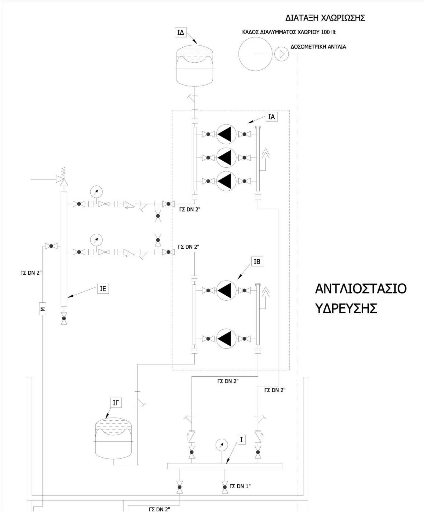
Λεπτομέρεια 4: Αντλιοστάσιο
