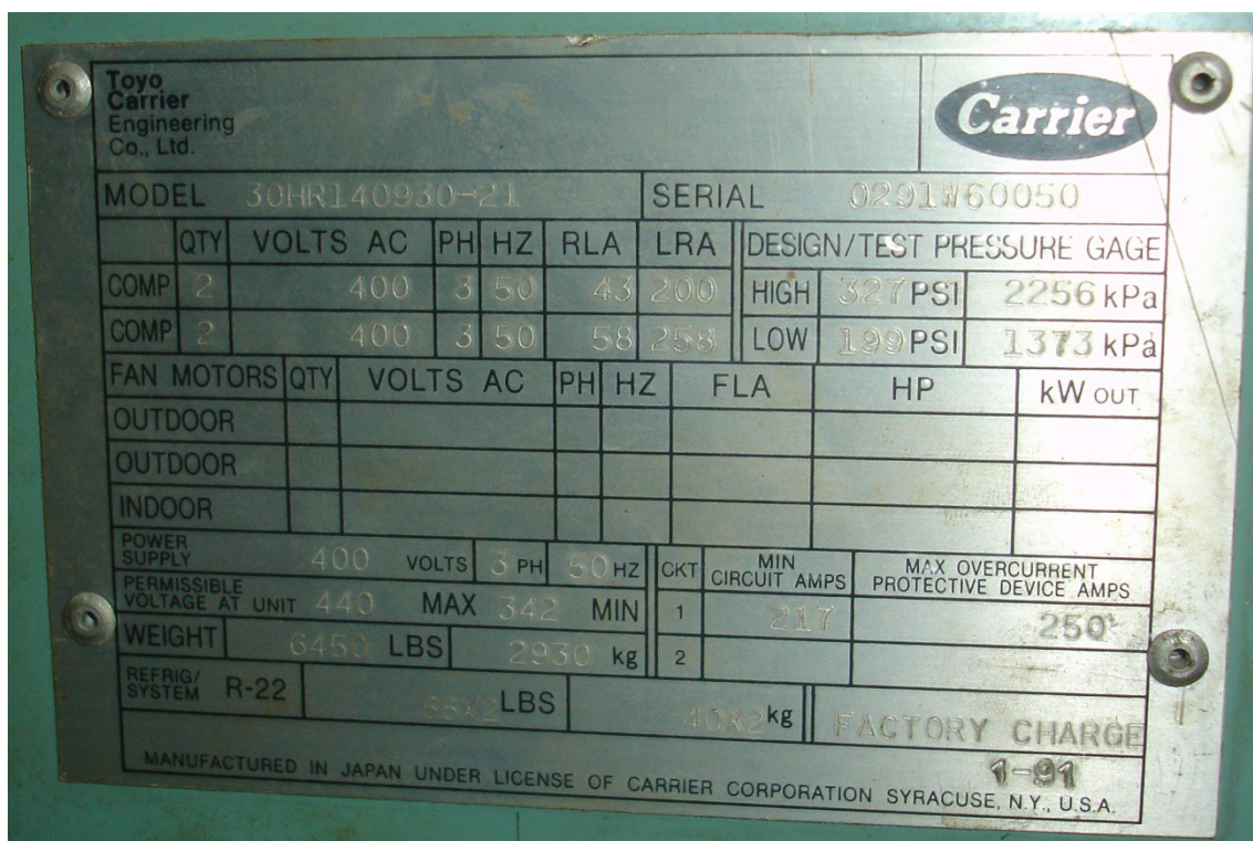
Φωτ 3: Στοιχεία υπάρχοντος ψυκτικού συγκροτήματος Carrier
