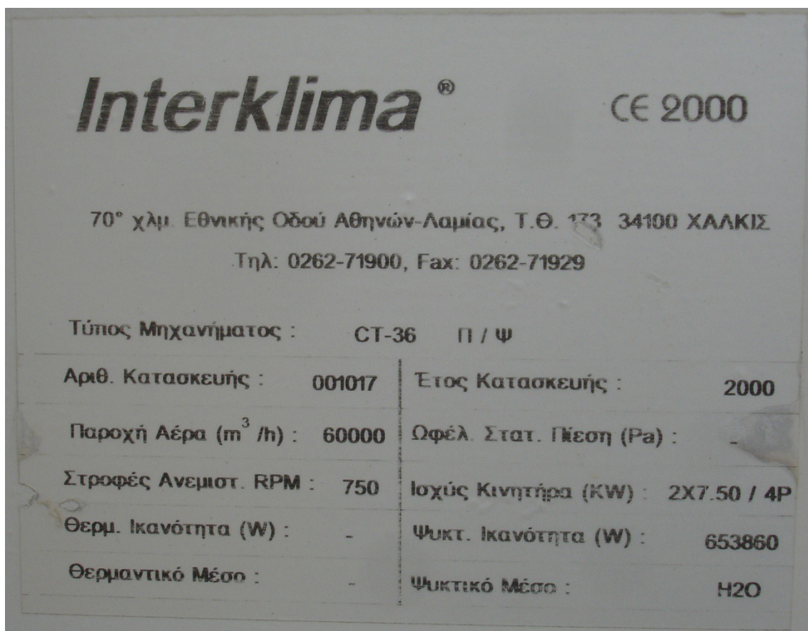
Φωτ 4: Στοιχεία υπάρχοντος πύργου ψύξης
