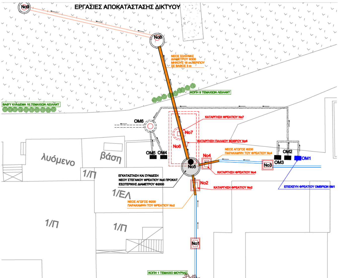
Σκαρίφημα 1: Εργασίες αποκατάστασης δικτύου
